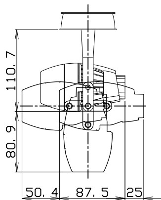
灯具可動時の最大寸法
